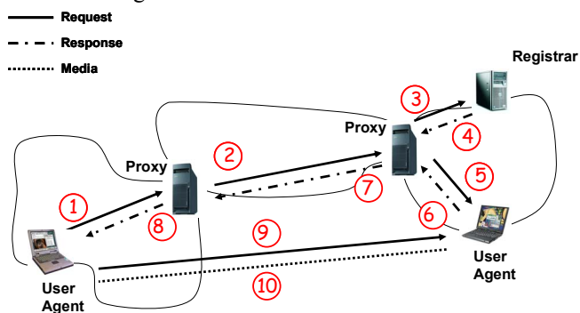
Fig. 1. Example SIP message flow
