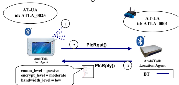
Fig. 3. BPS message flow
