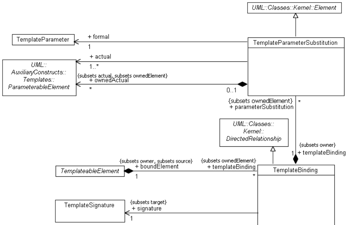
Figure 17.17 - Template parameters
