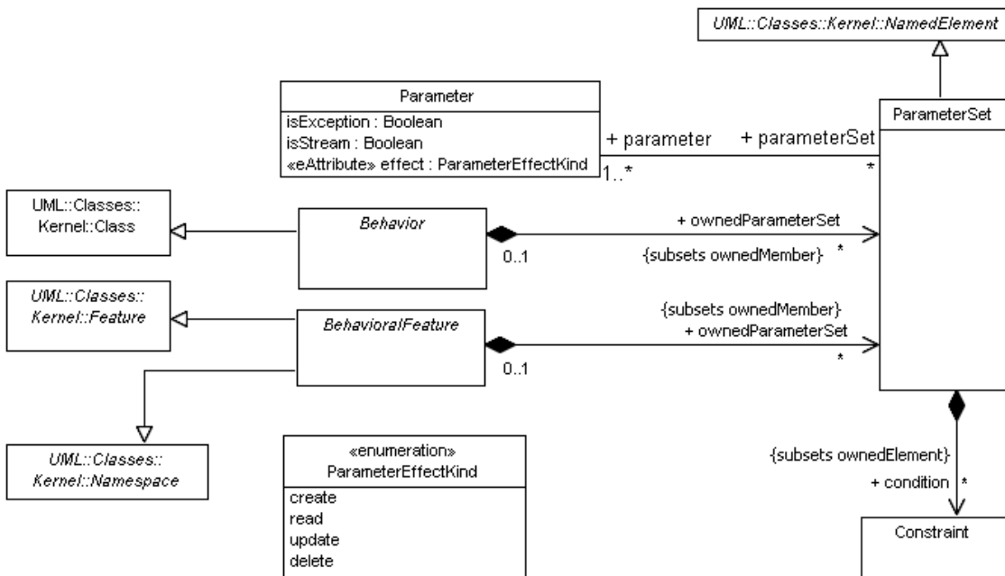
Figure 12.18 Parameter sets
